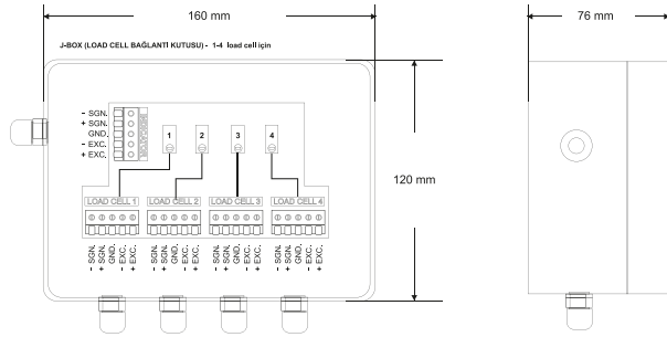
1-4 lü j box ölçüler ve bağlantı şeması
